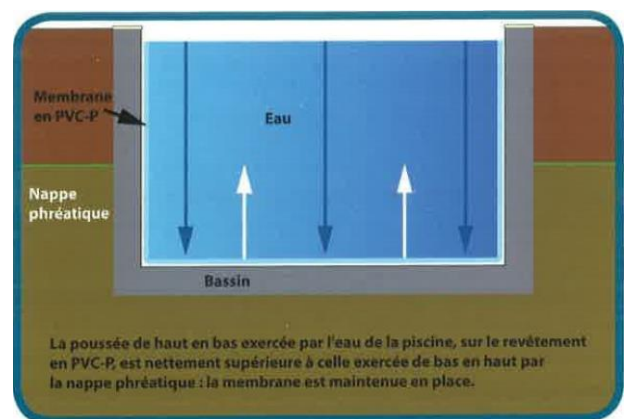
Le revêtement d'étanchéité reste plaqué, malgré la présence d'eau entre le bassin et la membrane en PVC-R
