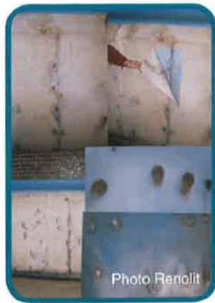
La formation de colonies de bactéries, entre la membrane et son support, a engendré des taches de sulfures métalliques, à la surface du revêtement.
