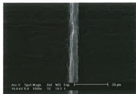
Après 2 ans, à pH 11 / 75°C
